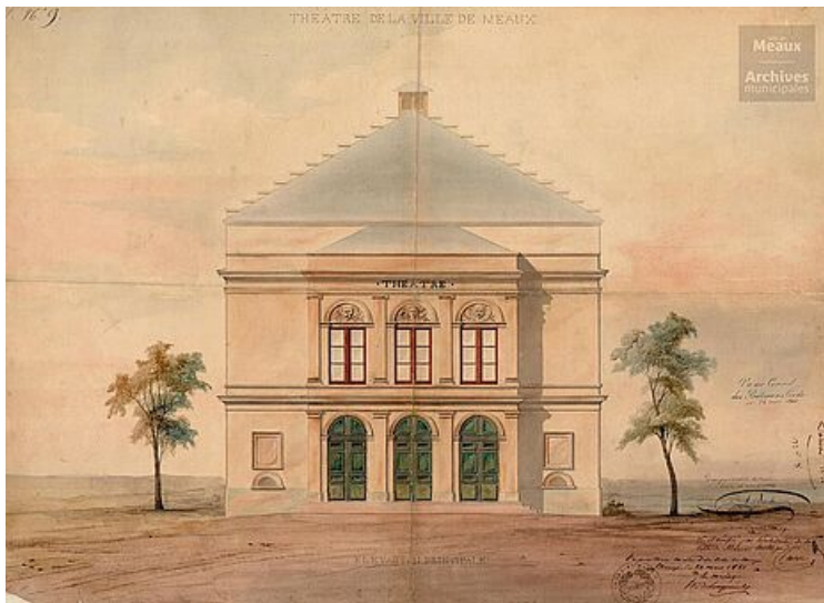
Alexandre BOURLA, Projet pour l'élévation de la façade principale , n°2F1173, 1840
