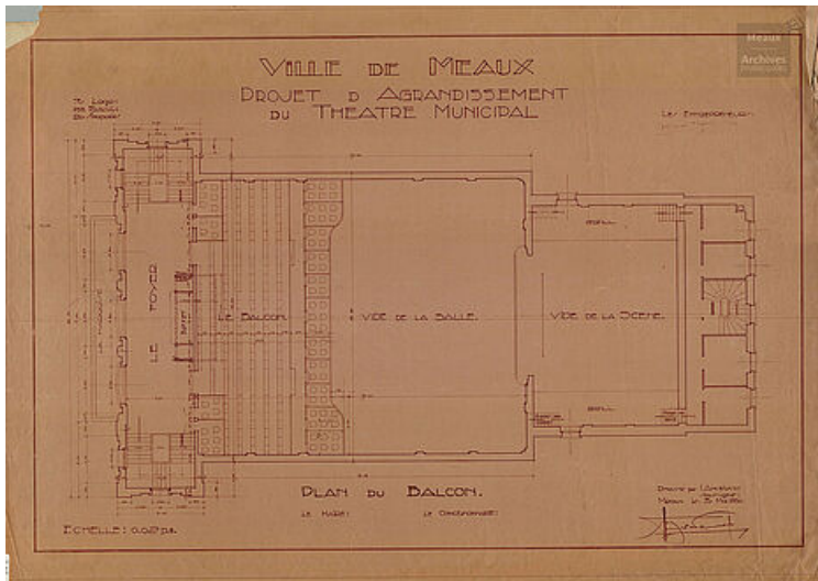
Henry FAUCHEUR, Projet d'agrandissement : plan du balcon, n°2F1733, 1934
