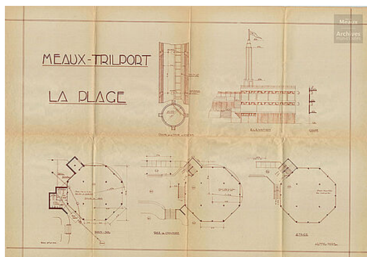
ODENT H., Elévation, coupe de la tour, sous-sol, rez de chaussée et étage, 4 O 26 (1), 1934
