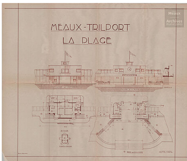
ODENT H., Elévation, plan et coupe, 4 O 26 (7), 1934
