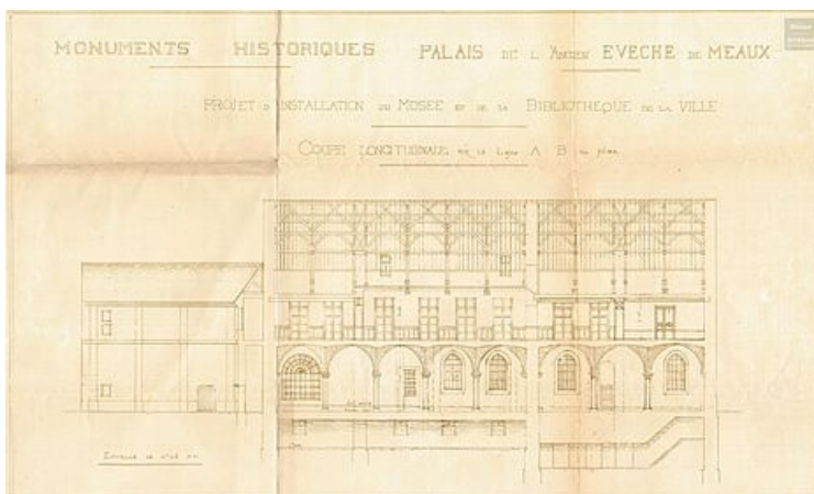
Palais de L'ancien Evêché de Meaux, Projet d'installation du Musée et de la Bibliothèque de la ville, Coupe longitudinale, 2F1838, (s.d.).
