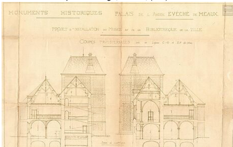
Palais de L'ancien Evêché de Meaux, Projet d'installation du Musée et de la Bibliothèque de la ville, Coupes transversales, 2F1837, (s.d.).
