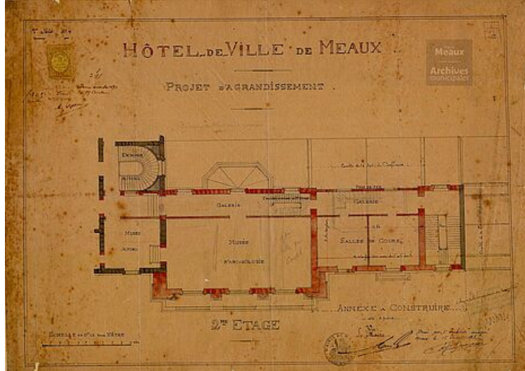
BOUDINAUD Auguste, Projet d'agrandissement : plan du deuxième étage, n° 2FI457, 1893
