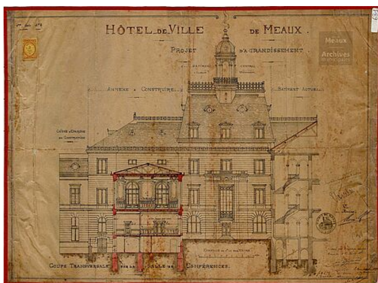
BOUDINAUD Auguste, Projet d'agrandissement : coupe transversale sur la Salle de Conférence, n° 2FI631, 1893
