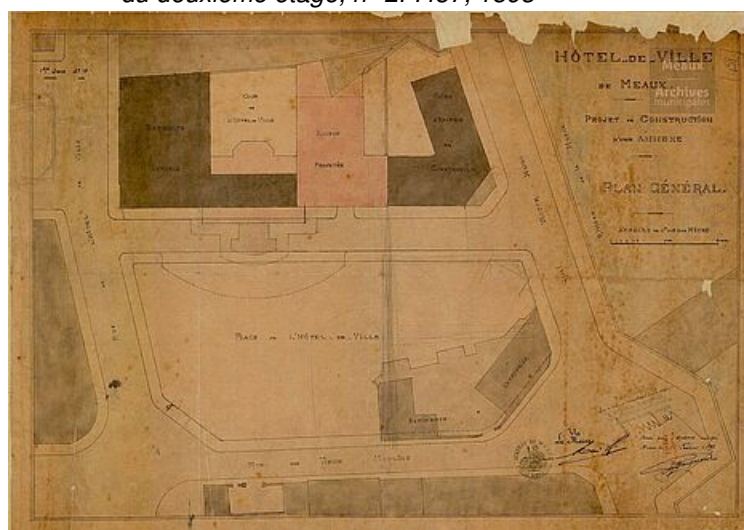
BOUDINAUD Auguste, Projet de construction d'une annexe : plan général, n° 2FI458, 1893
