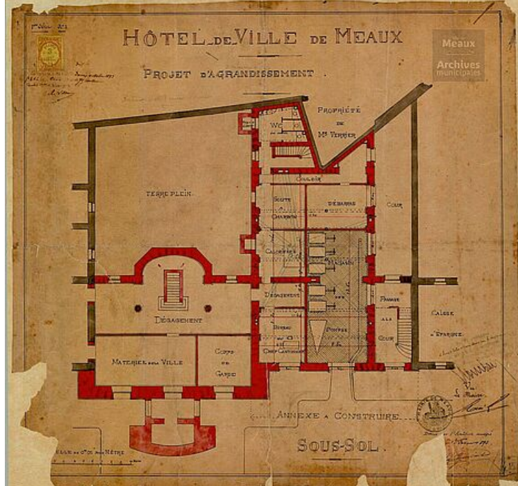
BOUDINAUD Auguste, Projet d'agrandissement - construction de l'annexe : plan du sous-sol, n° 2FI455, 1893
