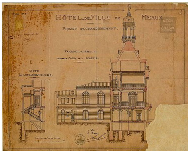
BOUDINAUD Auguste, Projet d'agrandissement: façade latérale, côté de la cour de la Mairie, coupe sur l'Escalier d'Honneur, n° 2FI456, 1893
