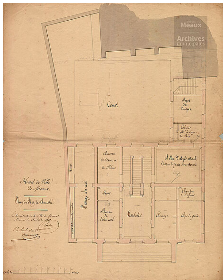
Pierre Didier Prosper Savard, Projet d'agrandissement : plan du rez-de chaussée, n° 2F1146, 1827
