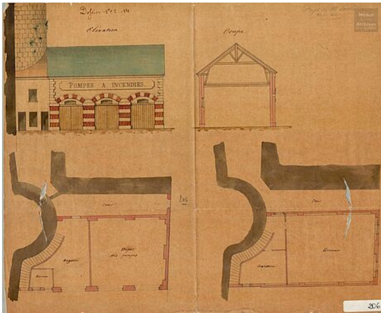
SAVARD Fils, Projet de construction d'un dépôt de Pompes à Incendie et d'un magasin, Elévation de la façade, Coupe, Plan du rez de chaussée et du 1er étage, 2FI206, (s.d.).
