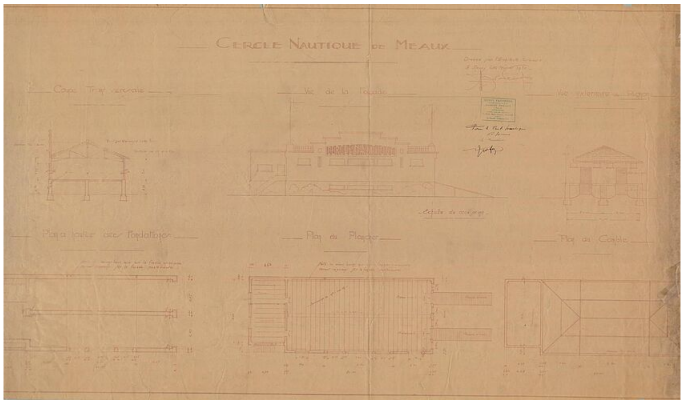
FAUCHEUR Henri, Cercle nautique de Meaux, coupe transversale plan à hauteur des fondations, plan du plancher, de la façade, vue extérieure du pignon, plan du comble, 1931
